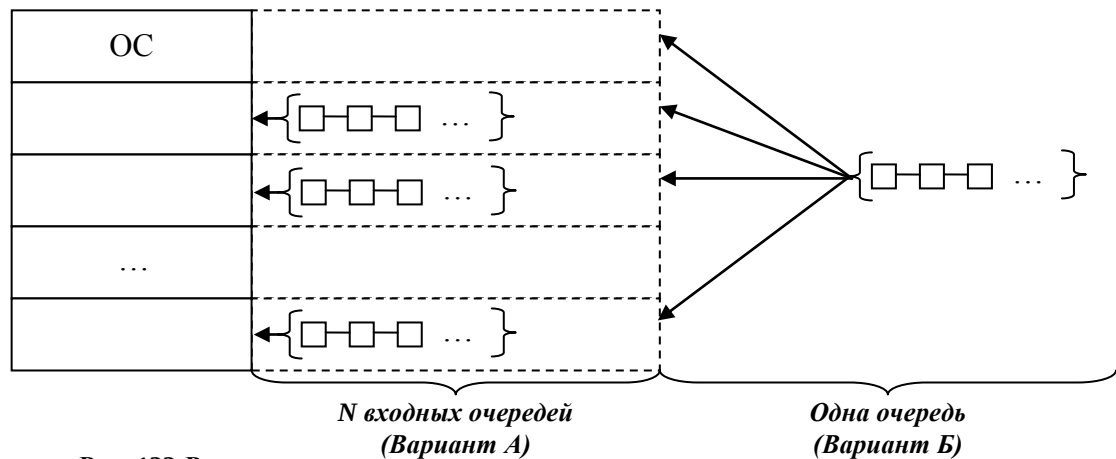
Рис. 132. Распределение неподвигаемыми разделами.
