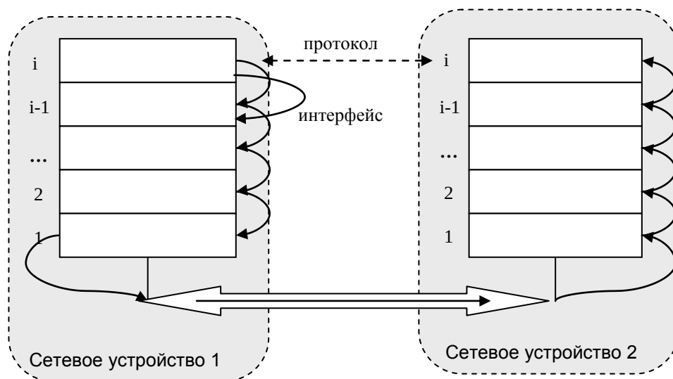
Рис. 67. Логическое взаимодействие сетевых устройств по i-ому протоколу.
