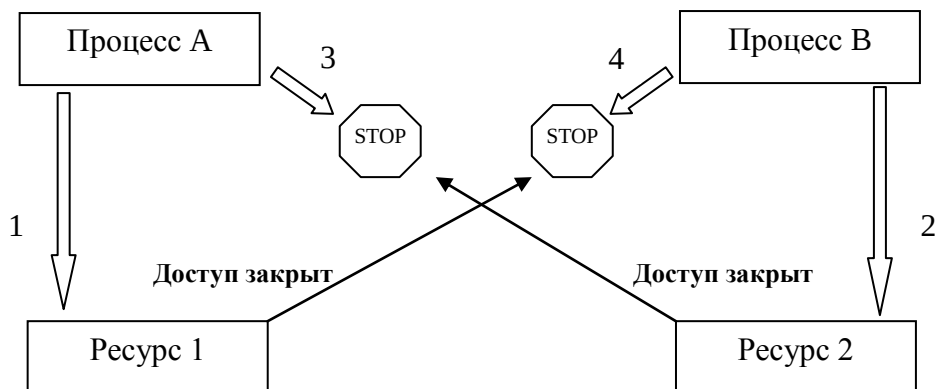
Рис. 92. Пример тупиковой ситуации (deadlock).
