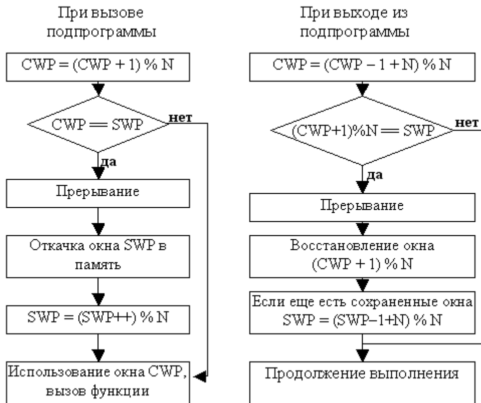
Рис. 51. Регистровые окна. Вход и выход из подпрограммы.
