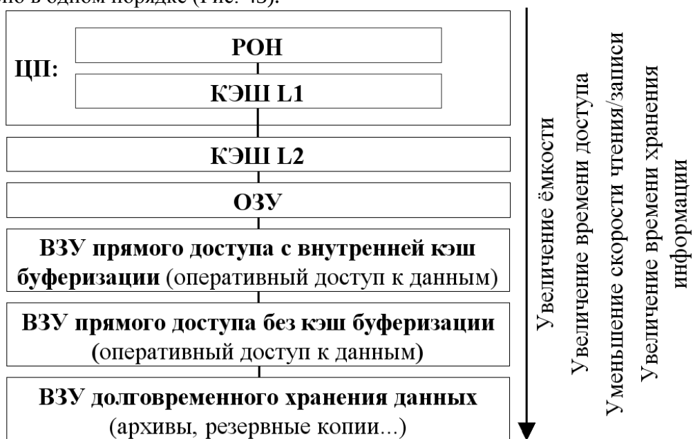
Рис. 43. Иерархия устройств хранения информации.
