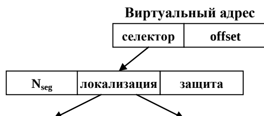
Рис. 142. Сегментно-страничное распределение. Упрощенная модель Intel.
