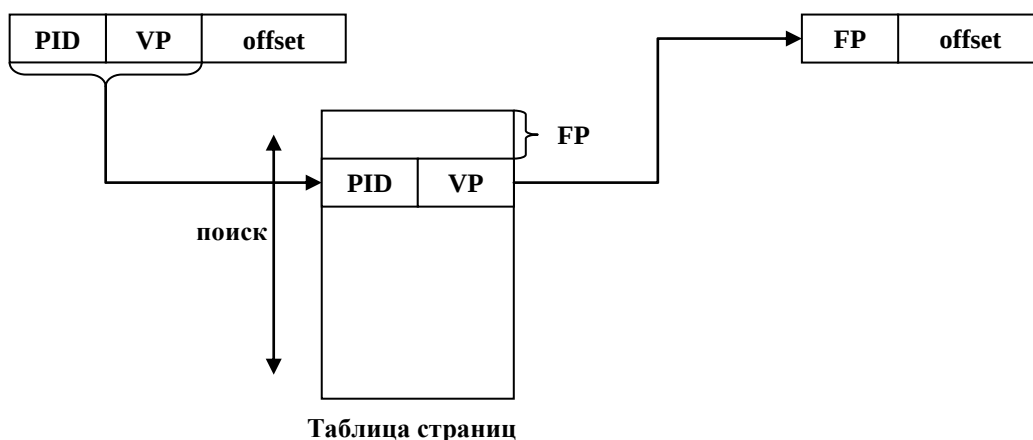
Рис. 139. Инвертированные таблицы страниц.
