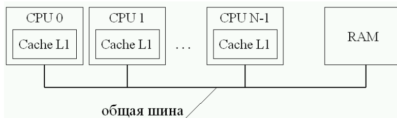
Рис. 60. Схема SMP-системы.
