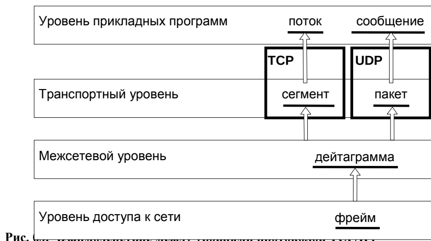
Рис. 1. Взаимодействие между уровнями протокола TCP/IP.
