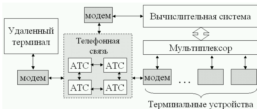
Рис. 63. Структура терминального комплекса.
