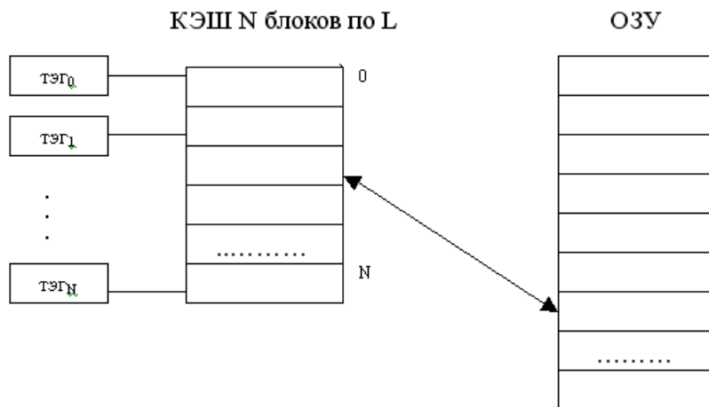
Рис. 28. Общая схема работы КЭШа.
