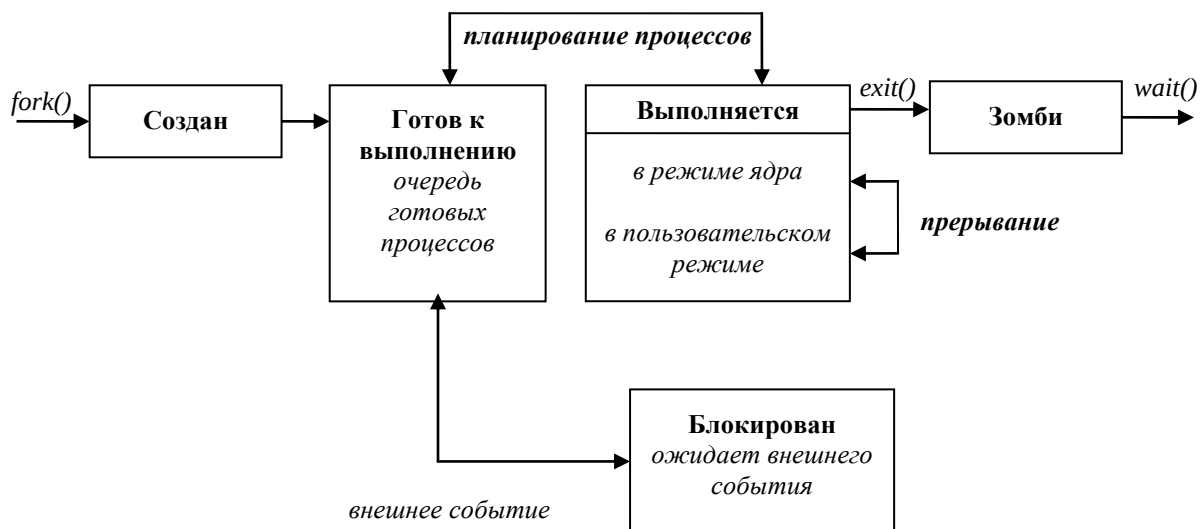
Рис. 87. Жизненный цикл процессов ОС Unix.
